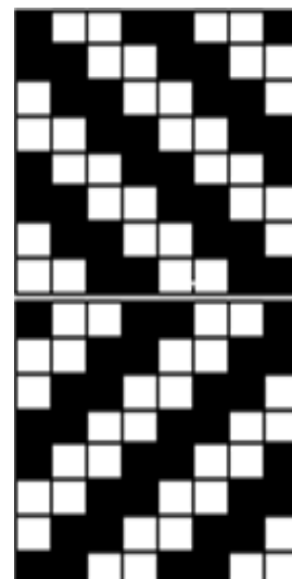
Armure sergé sans envers de 4 ou armure croisé de 4
