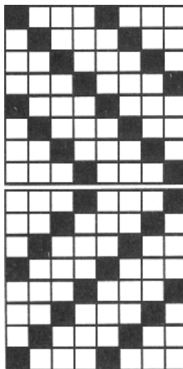
Armure sergé de 4
