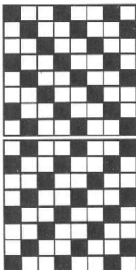
Armure sergé de 3
